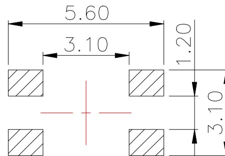
PCB.焊接图
